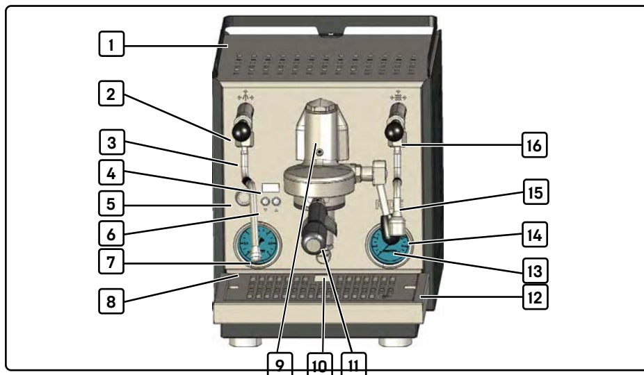
Fig. 1 Structure et composants
